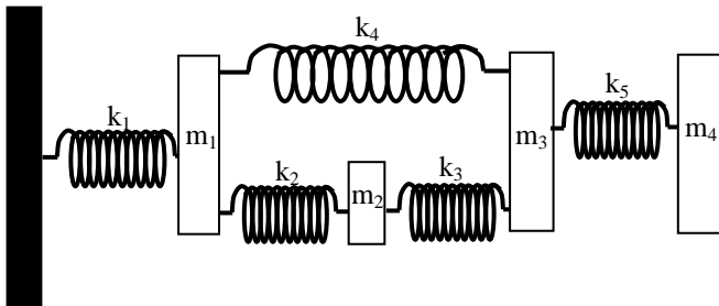
Gambar 1.1 : Tinjauan sistem empat massa dan lima pegas (Sumber: Dokumen pribadi)
