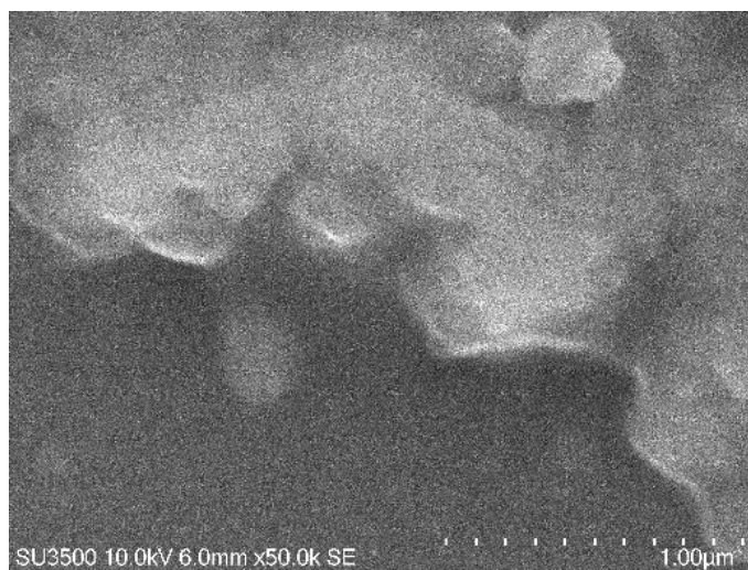
Morfologi yang diamati dengan SEM 50,0kV Gambar 2. Morfologi Partikel dengan SEM
