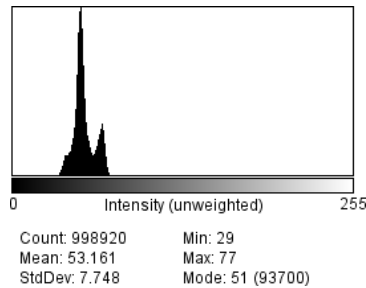
Gambar 7 Hasil Citra Radiografi grafik histogram software Image-J dengan Faktor ekspos 50 kV, 60 kV , 70 kV, jarak 100 cm dan 10 mAs
