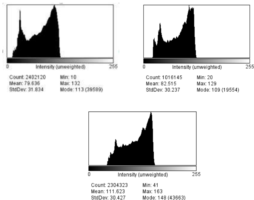
Gambar 8 Hasil Citra Radiografi grafik histogram software Image-J dengan Faktor ekspos 90 kV, 100 kV, 110 kV, jarak 100 cm dan 10 mAs
