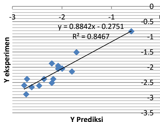
Gambar 2. Grafik Linear antar nilai Log (1/IC 50 ) eksperimen dengan Log (1/IC 50 ) prediksi Persamaan 18
