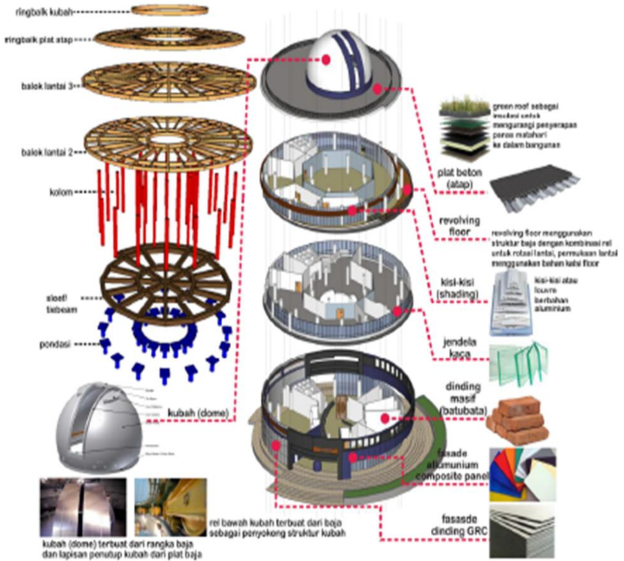
Gambar. 10: Konsep Struktur dan Material Gedung Utama (Observatorium) Sumber: Olah Desain, 2015
