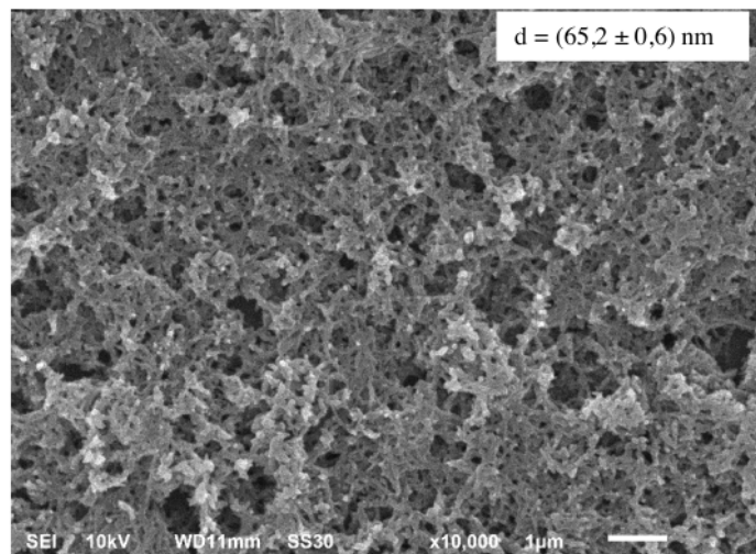
Gambar 3. Hasil SEM dengan konsentrasi HCl 0,6 M
