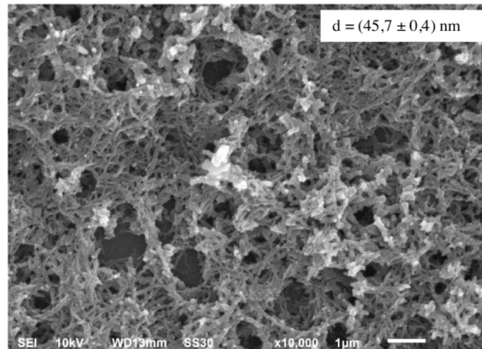
Gambar 5. Hasil SEM dengan konsentrasi HCl 3 M
