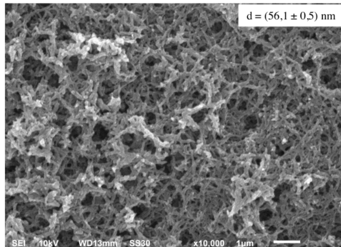
Gambar 4. Hasil SEM dengan konsentrasi HCl 1,8 M
